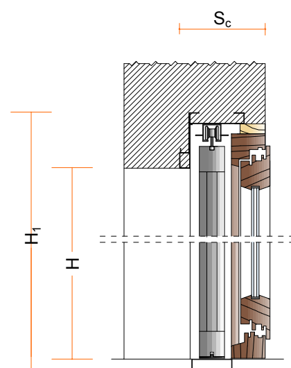
SEZIONE VERTICALE
