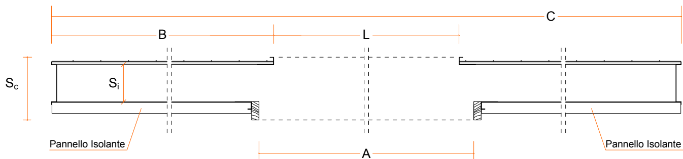
SEZIONE ORIZZONTALE
